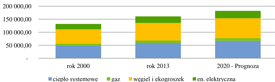
Rysunek 29. Emisja generowana przez pokrycie zapotrzebowania na energię cieplną dla gminy Brańszczyk na lata 2000, 2013 oraz prognoza na 2020 rok
