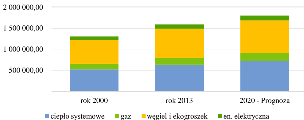
Rysunek 28. Struktura pokrycia zapotrzebowania na energię ciepłą na lata 2000, 2013 oraz prognoza na 2020 rok
